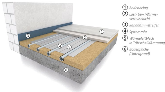
Abbildung 9: Praxisbeispiel Bodenaufbau – Trockensystem (Registerbauweise)
