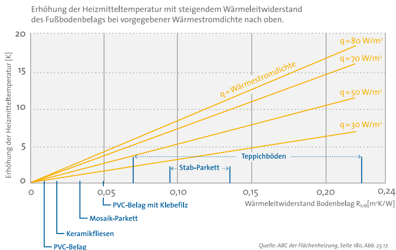
Abbildung 15: Notwendige Erhöhung der Heizmitteltemperatur in Abhängigkeit unterschiedlicher Wärmeleitwiderstände des Bodenbelags
