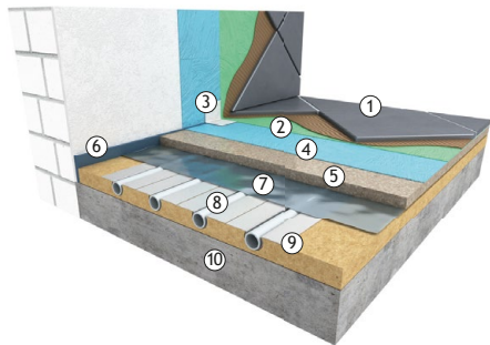
Abbildung 14: Abdichtung gegen Oberflächenwasser (Sanitärbereiche)
