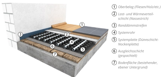
Abbildung 12: Ausgleichsspachtel auf einem bestehenden Bodenbelag
