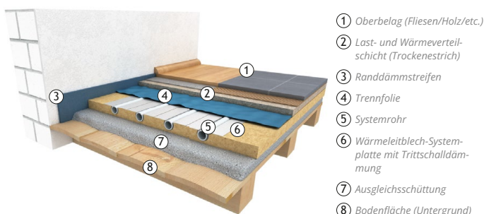
Abbildung 11: Ausgleichsschüttung auf einem bestehenden Dielenboden mit Trockensystem Registerbauweise
