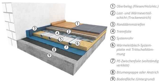
Abbildung 13: Bodenaufbau mit Abdichtung gegen aufsteigende Feuchte (Abdichtung gegen Bodenfeuchte)
